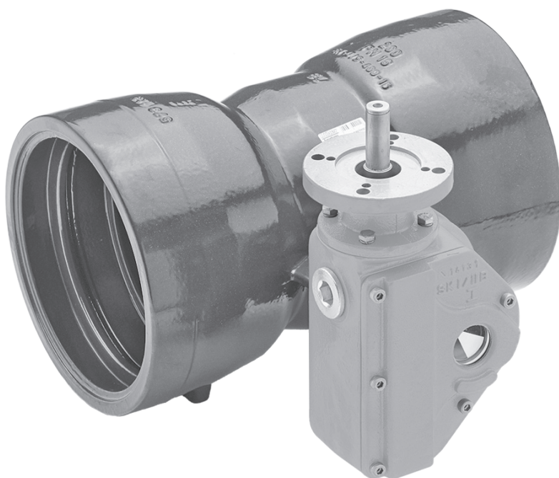
Valvola a farfalla con volantino/guarnizione di posa/attuatore elettrico
