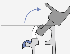
Ouverture à 130°
