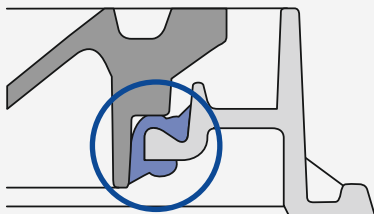
Insert élastomère
